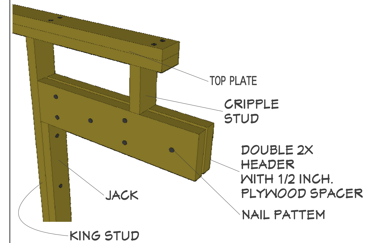
DOOR HEADER DETAIL S-4
